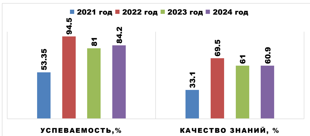
Рисунок 3. Мониторинг успеваемости
